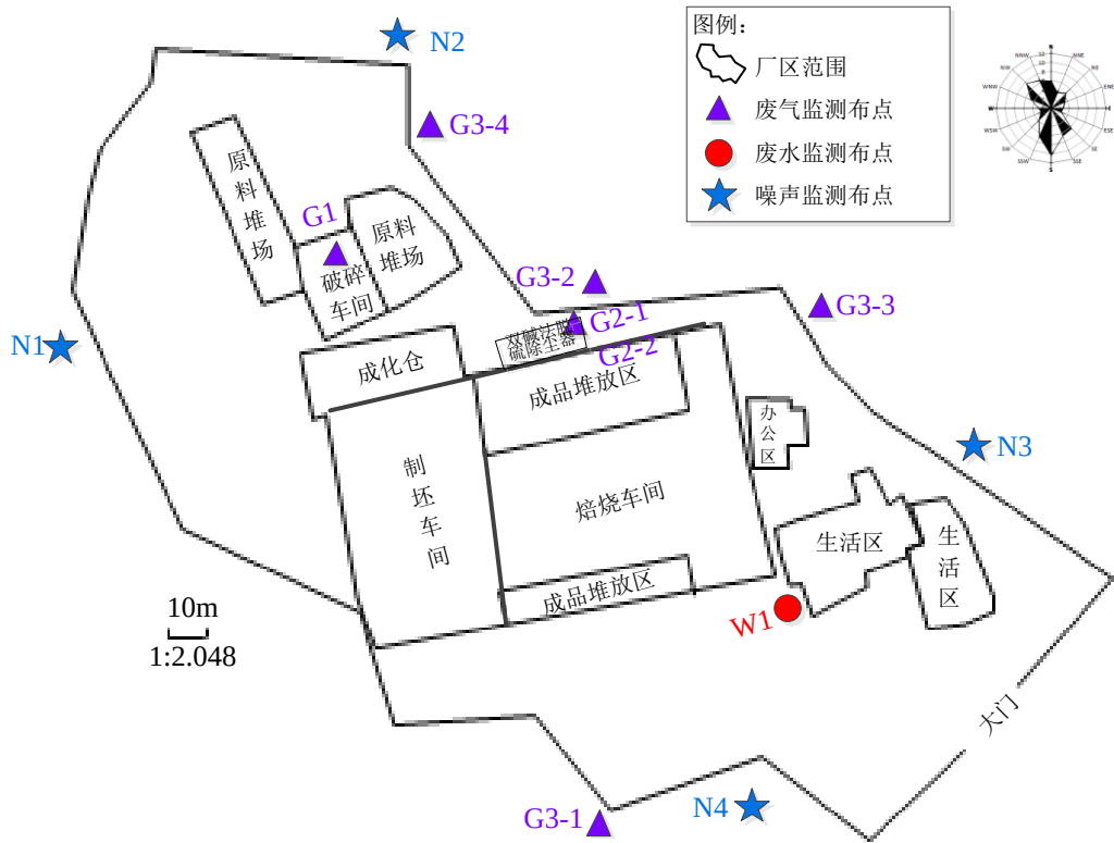
图 7.3-1 废气、废水、噪声监测布点图
