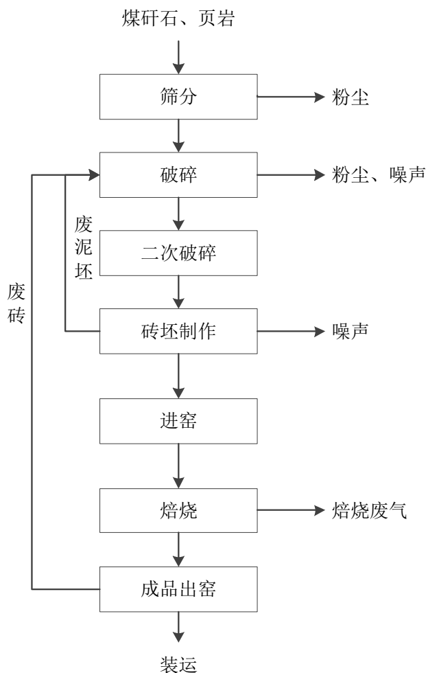
图 3.3-1 本项目生产工艺及产污节点图
