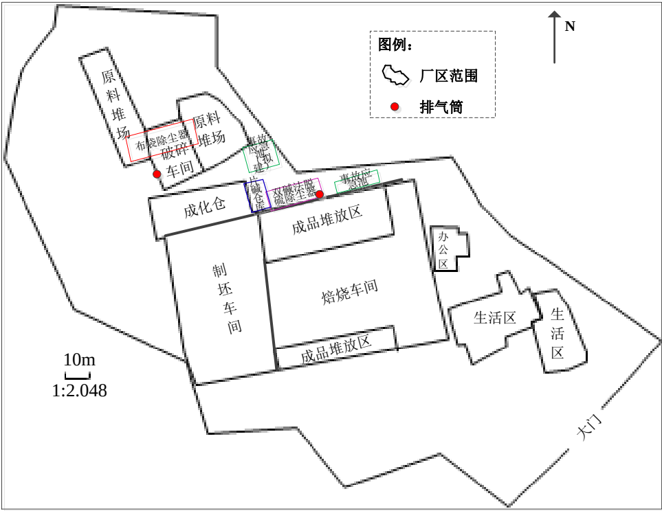
图 3.2-3 厂区平面布置图
