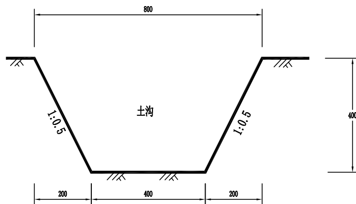
规划排灌土沟 1:10
