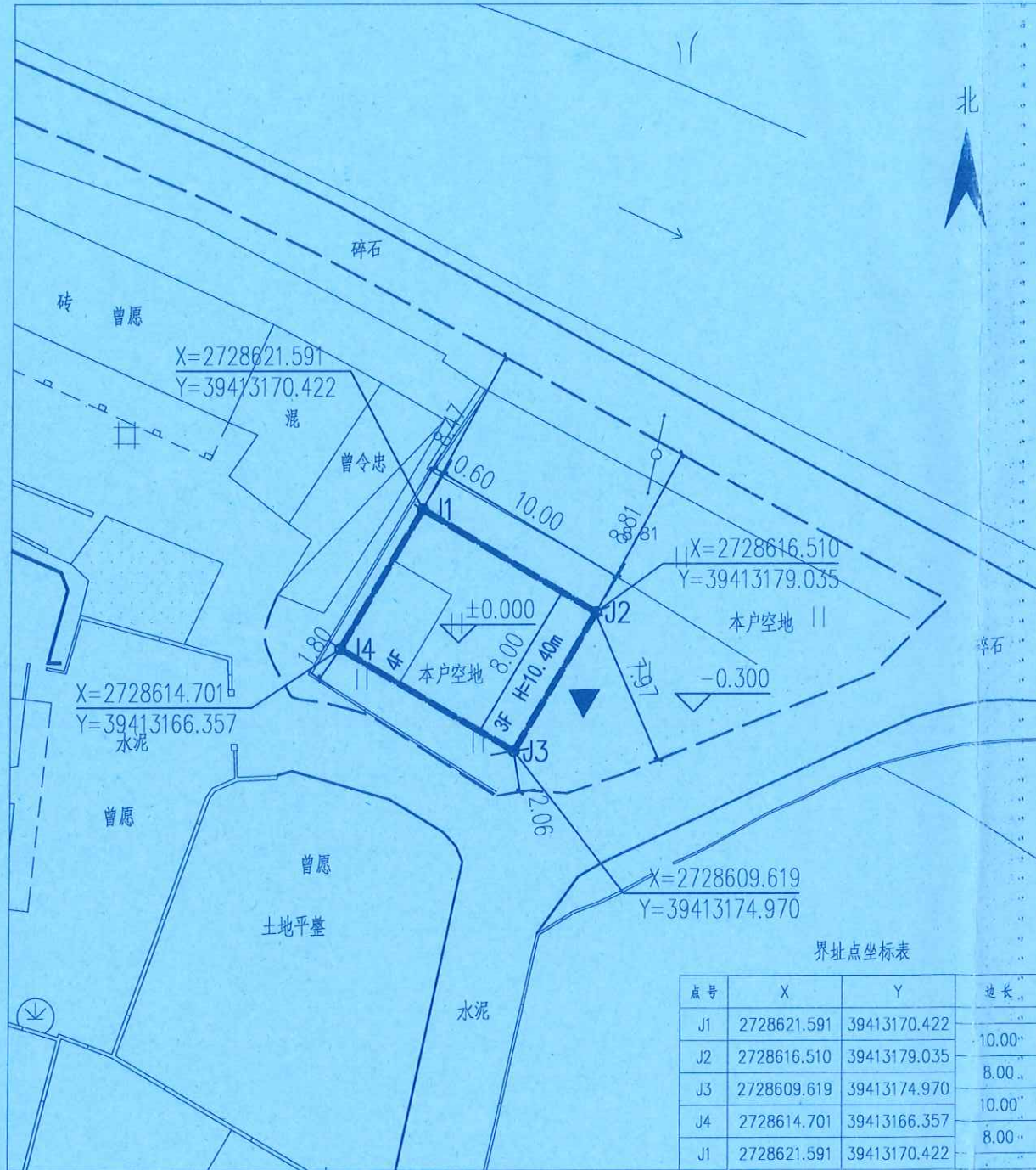
刘辉月【蕉岭县长潭镇埗垣村红山小组】房屋总平面图
