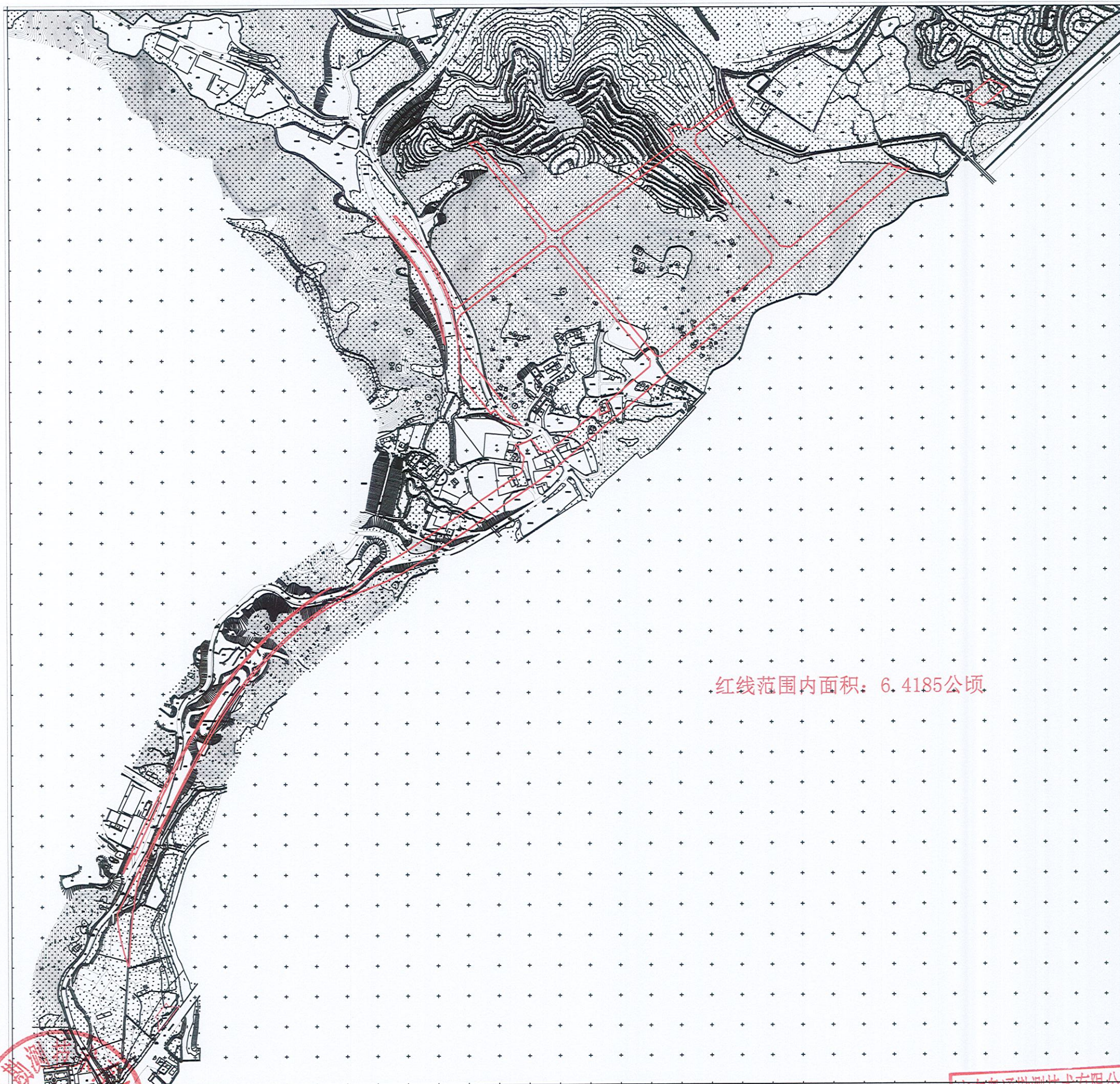
蕉岭县2022年度第八批次城镇建设用地勘测定界图（二）
